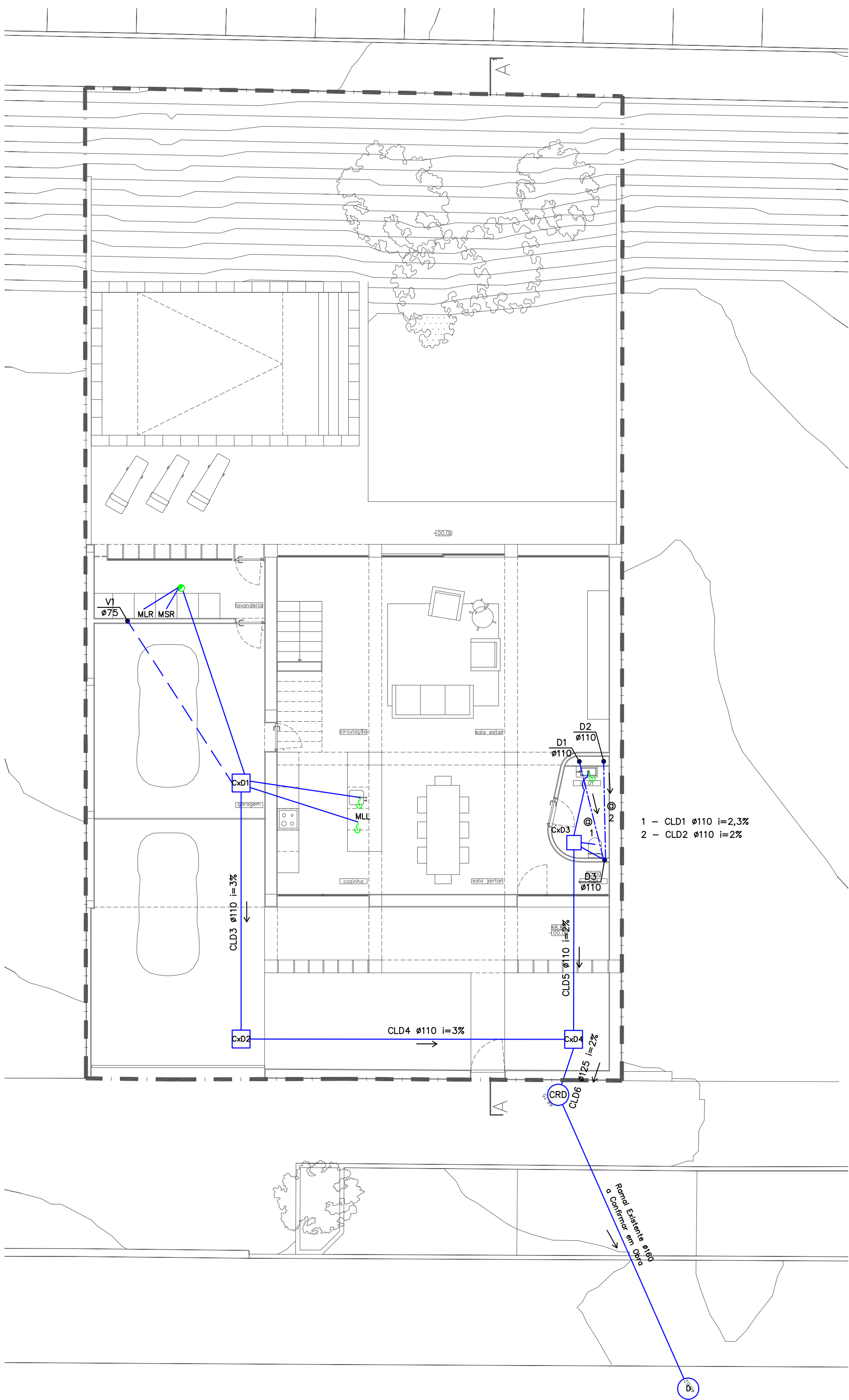
PLANTA DO PISO 0
