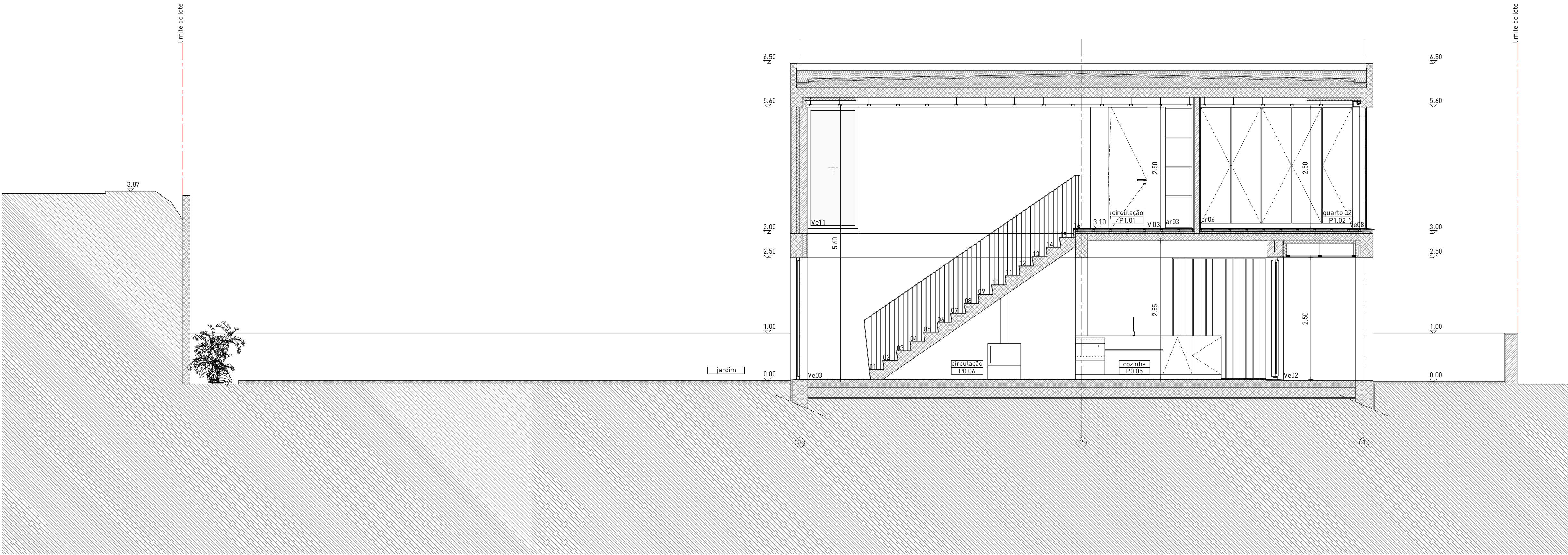
CORTE LONGITUDINAL DD'
