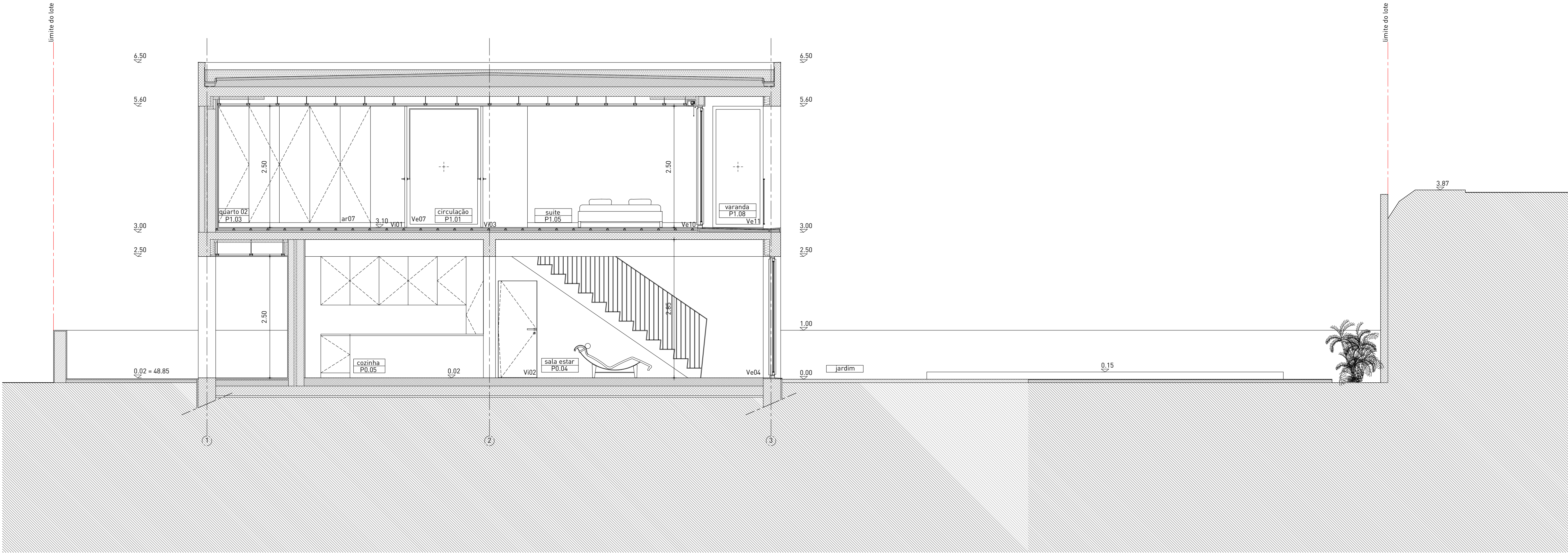
CORTE LONGITUDINAL AA'
