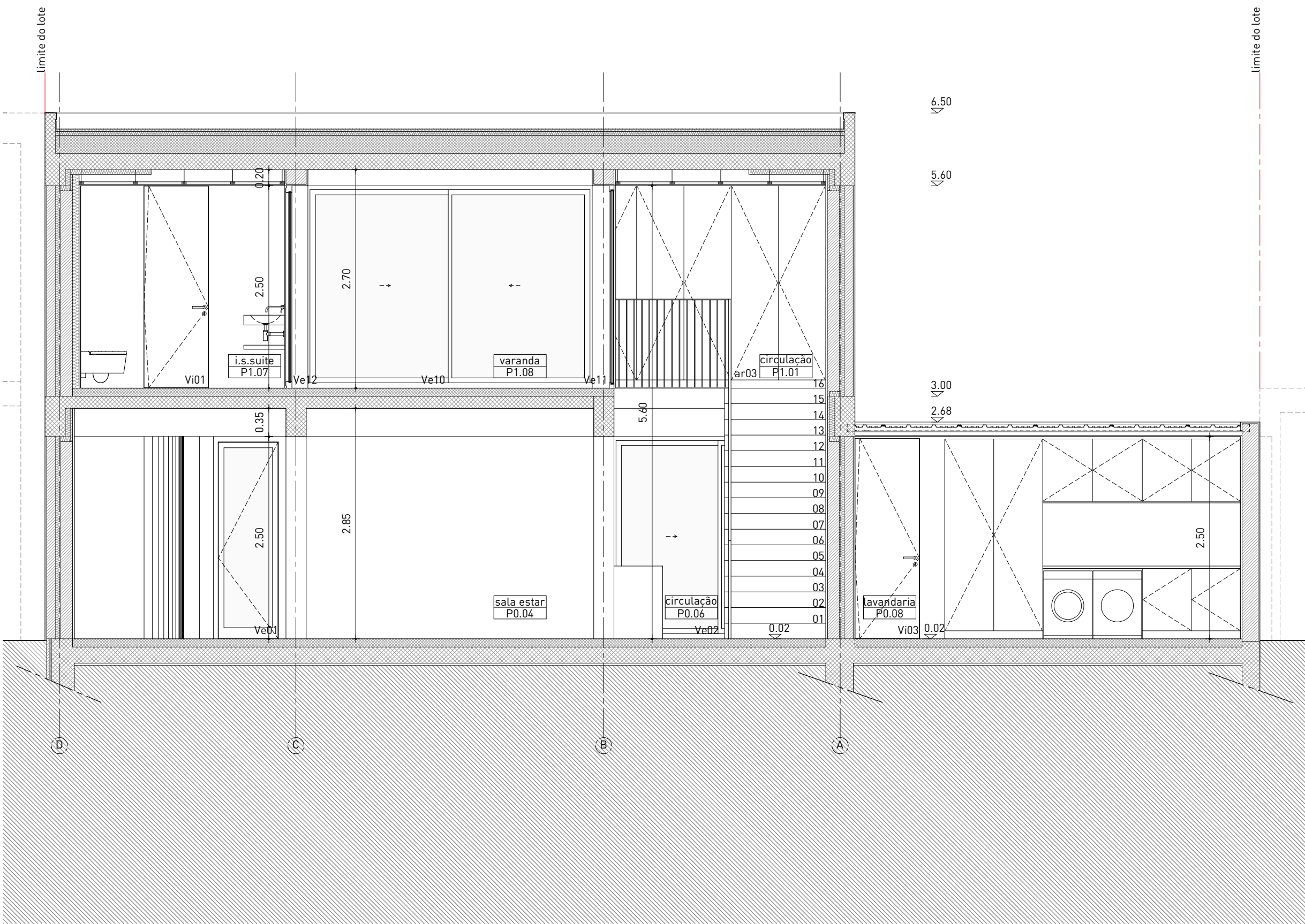
CORTE TRANSVERSAL CC'
