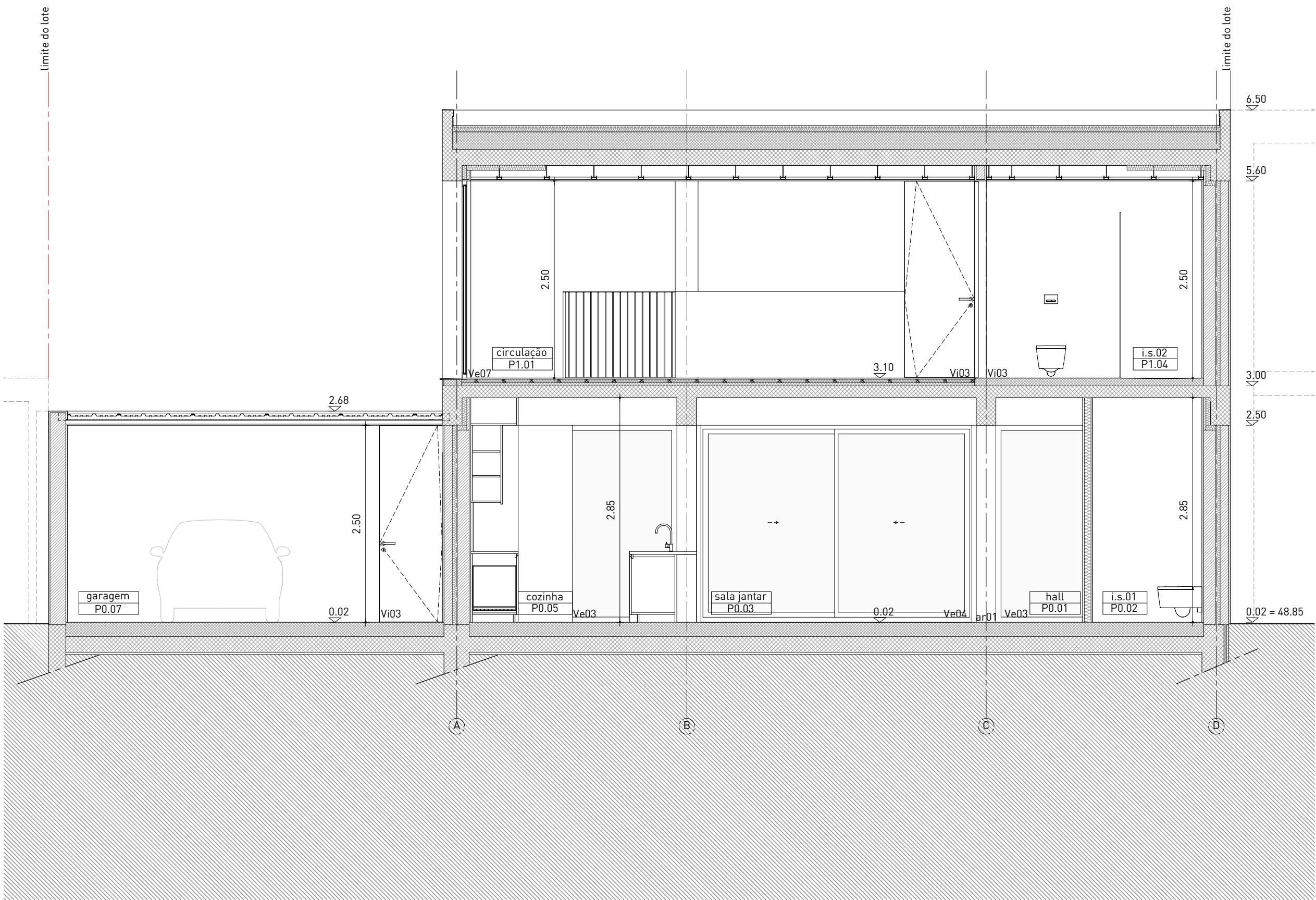
CORTE TRANSVERSAL BB'
